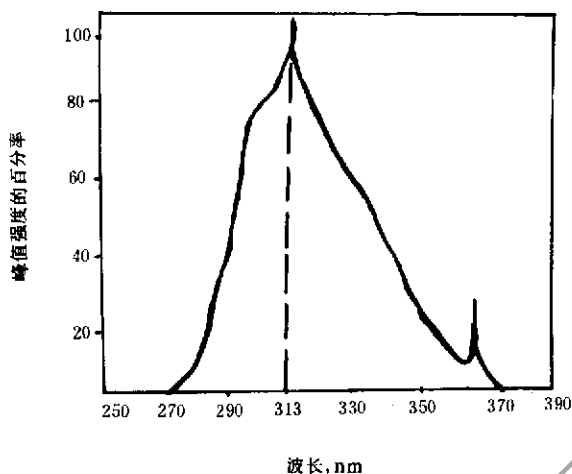
图3 UV-B 荧光紫外灯的相对分光光谱辐照度
