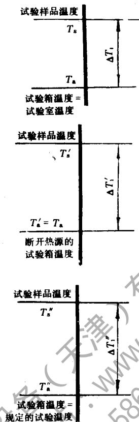
图 2 试验 Bd 方法 A 有强迫空气循环时试验样品的温度状况的图示
