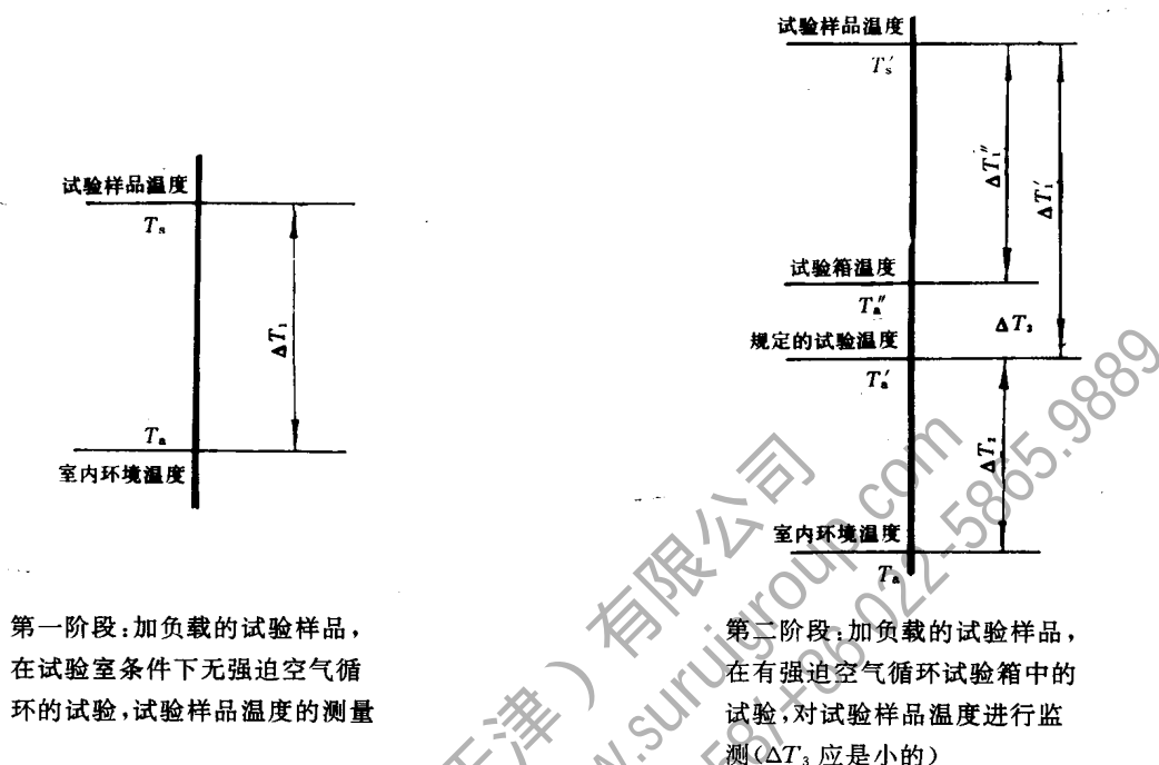
图 1 试验 Bc 和 Bd 中方法 B 有强迫空气循环、试验样品试验时试验温度情况的图示
