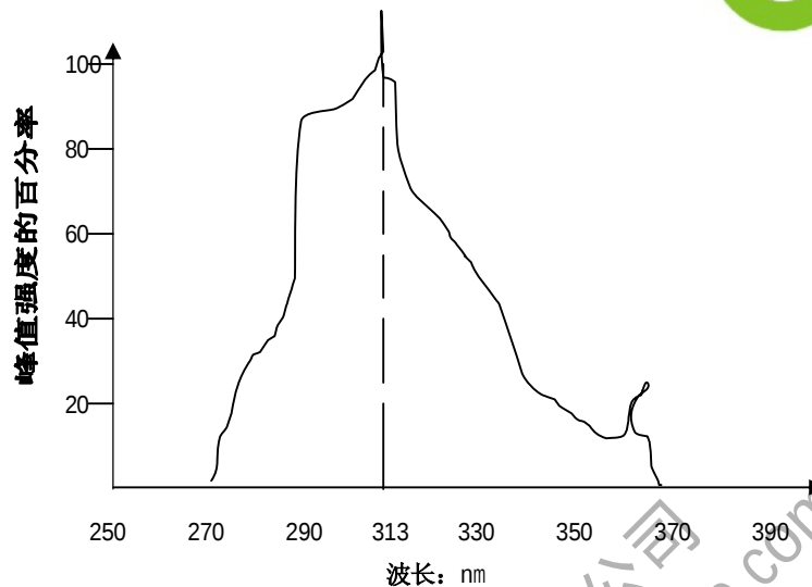
图3 UV-B 荧光紫外灯的相对分光光谱辐照度
