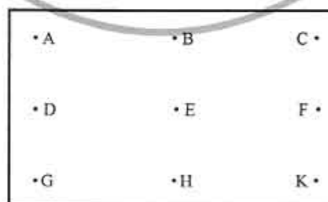
图 4 试验设备容积大于 2 \text{ m}^3 时盐雾沉降率测量点布放位置
