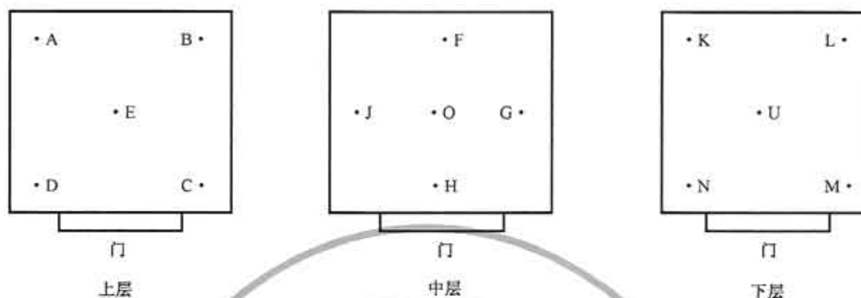
图 2 试验设备容积大于 2 \text{ m}^3 时温度测量点布放位置
