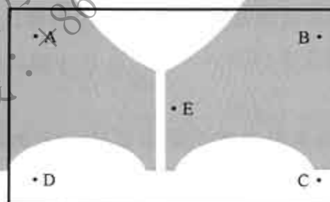
图 3 试验设备容积小于或等于 2 \text{ m}^3 时盐雾沉降率测量点布放位置
