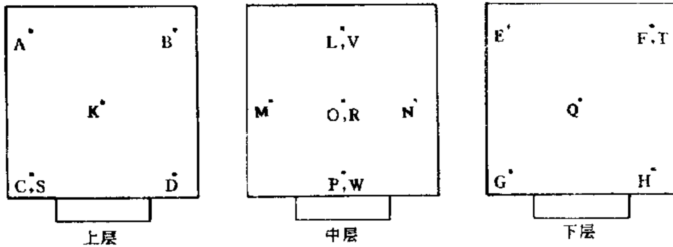
图2 容积大于 2\text{m}^3 的试验箱(室)温湿度测量点布置图
