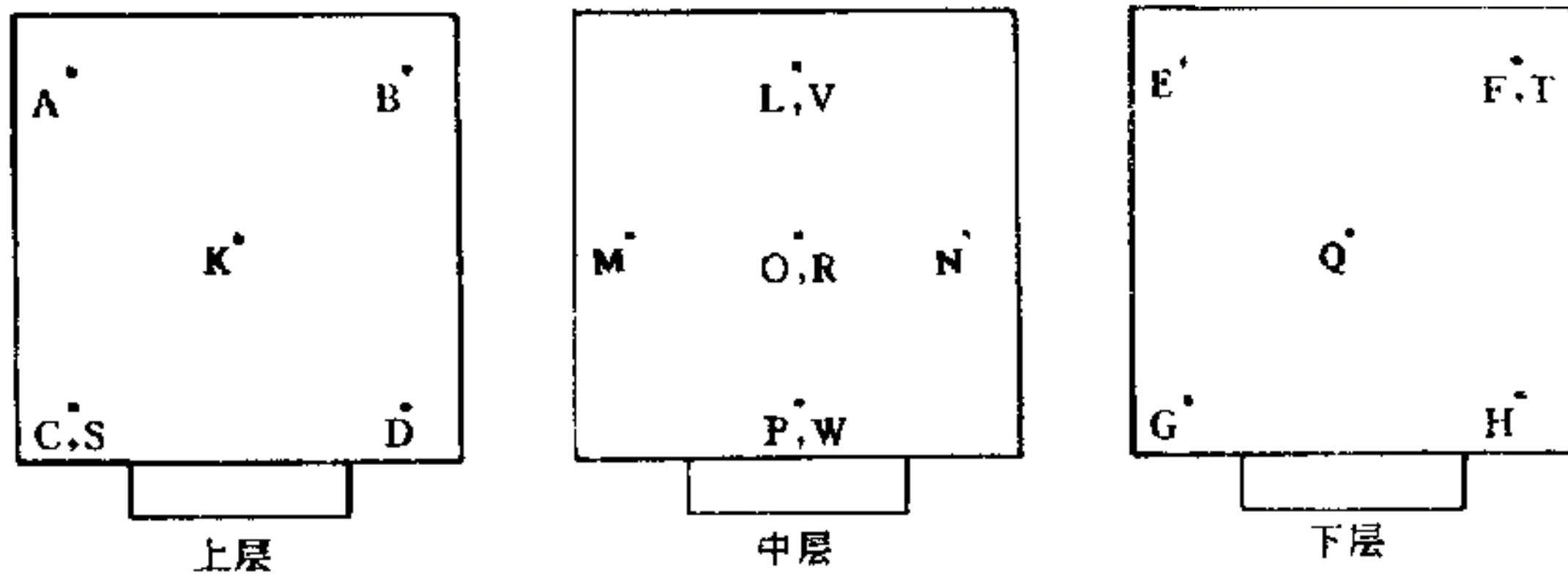
图2 容积大于 2m 3 的试验箱(室)温湿度测量点布置图
